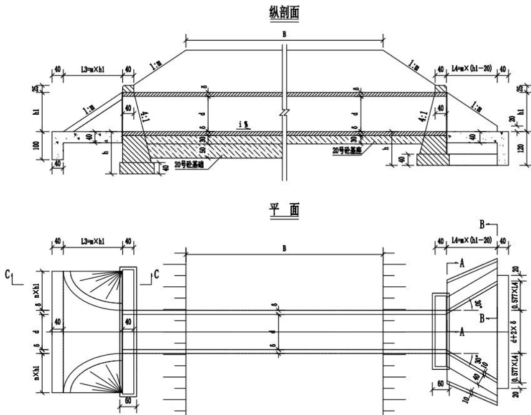
图 2.1-10 涵洞设计图
