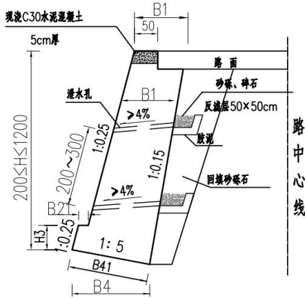
图 2.1-6 挡墙设计图 (1)
