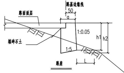
图 2.1-7 挡墙设计图 (2)
