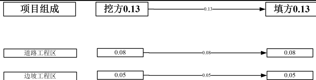
图 2.4-1 土石方流向框图 (单位: 万 m 3 )
