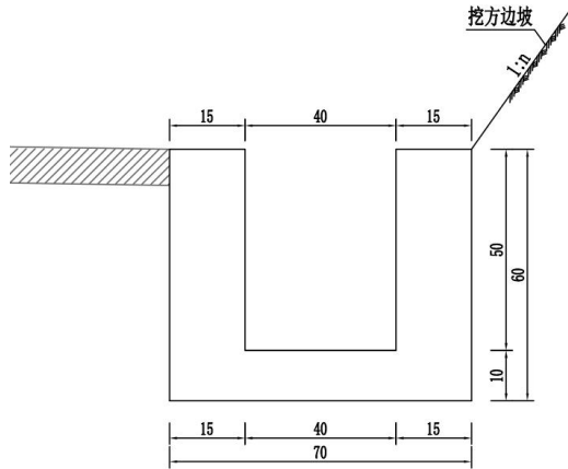
图 2.1-8 混凝土边沟设计图
