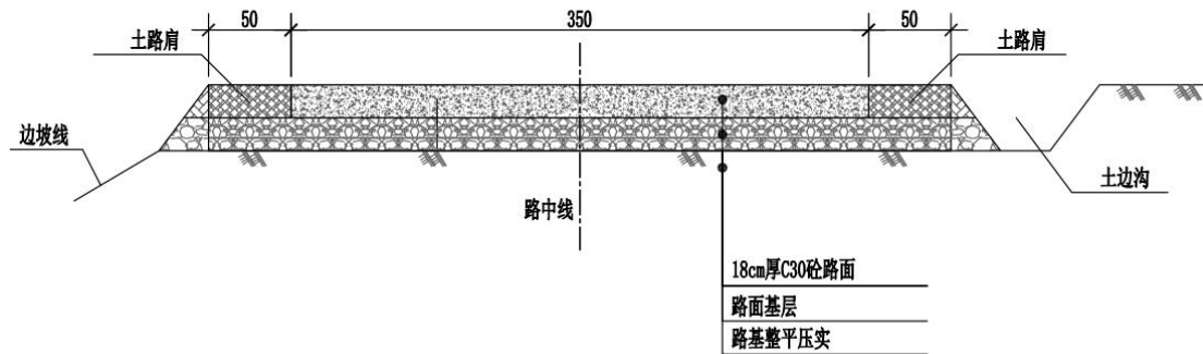
图 2.1-5 路基横断面图
